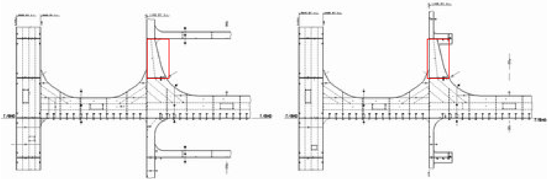
STRINGER PLAN I.W.O T/BHD
